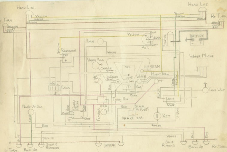
SCHEMA DE CABLAGE DE LA «MEHARI»
